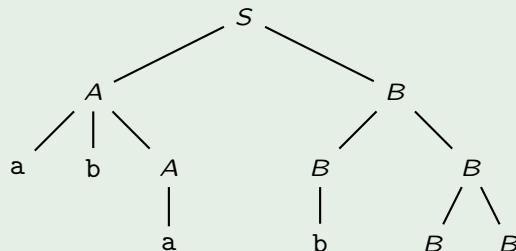
Ableitungsbaum von ababbb:
