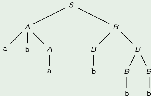
Ableitungsbaum von ababbb:
