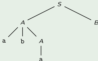
Ableitungsbaum von ababbb:
