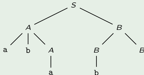
Ableitungsbaum von ababbb:
